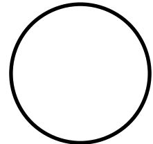
Kreis
