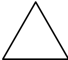
Dreieck
