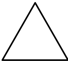
Dreieck
