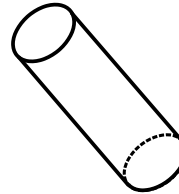
Zylinder
