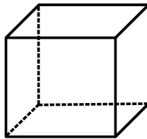
Würfel
