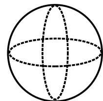
Kugel
