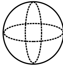
Kugel
