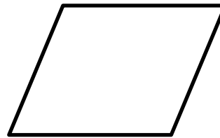
Parallelogramm
