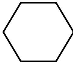
Sechseck
