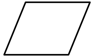
Parallelogramm
