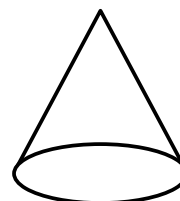
Kegel
