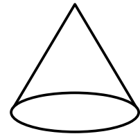
Kegel
