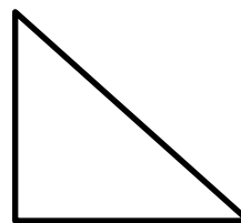
Dreieck
