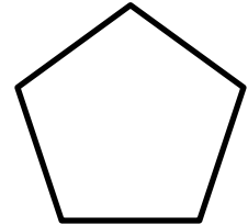
Fünfeck
