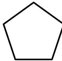
Fünfeck
