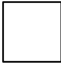
Quadrat
